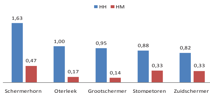
HH en HM afgezet tegen inwonersaantallen
