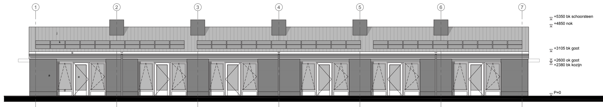
gevelaanzicht 03
