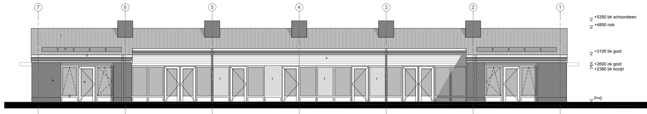
gevelaanzicht 01
