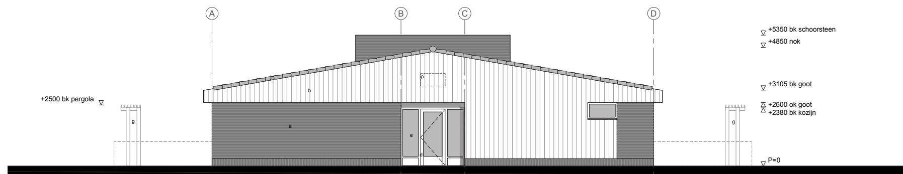
gevelaanzicht 02
