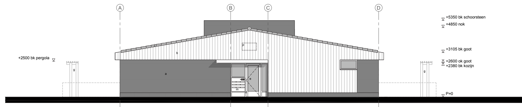
gevelaanzicht 02
