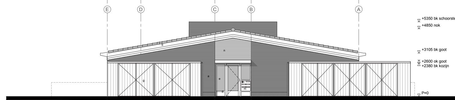
gevelaanzicht 04
