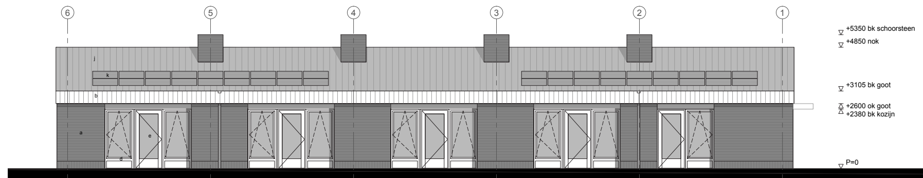
gevelaanzicht 01
