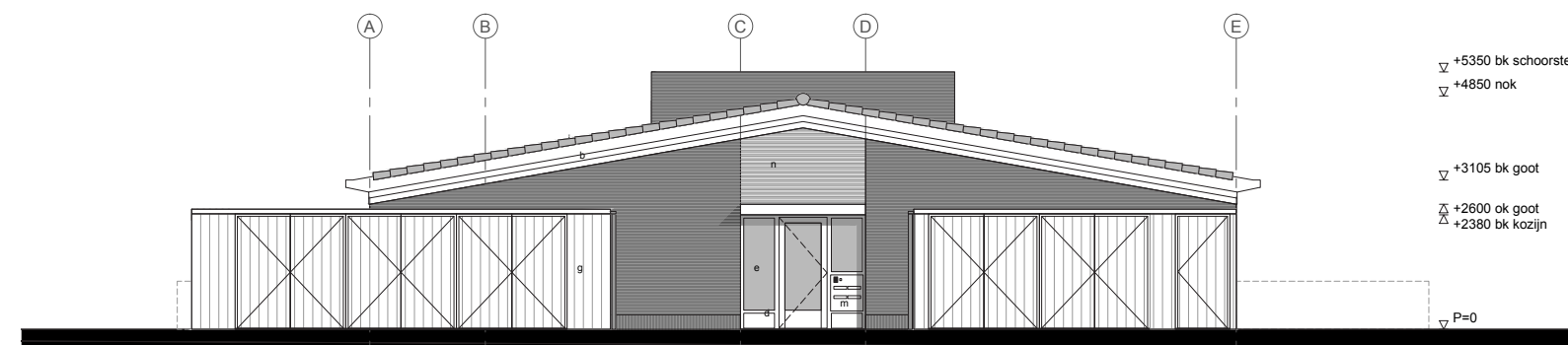
gevelaanzicht 02
