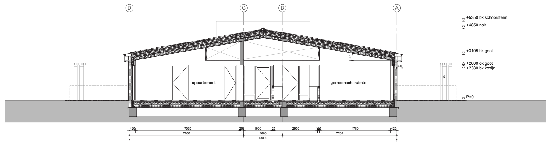
doorsnede A-A
